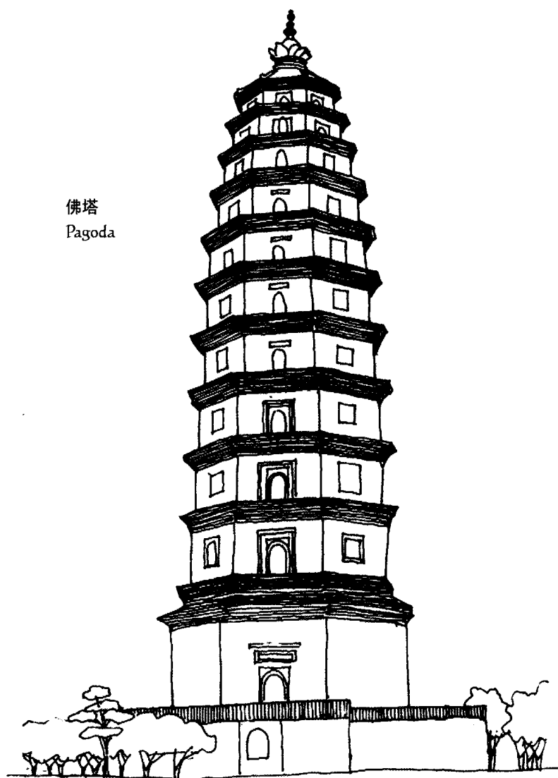
图 1-3 河北定县料敌塔（北宋，1001—1055 年）
