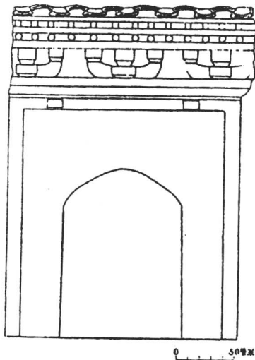
图二 M5 仿木门楼正视图
