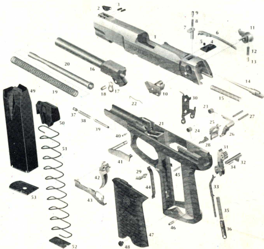
美国9mm鲁格P89手枪分解图
