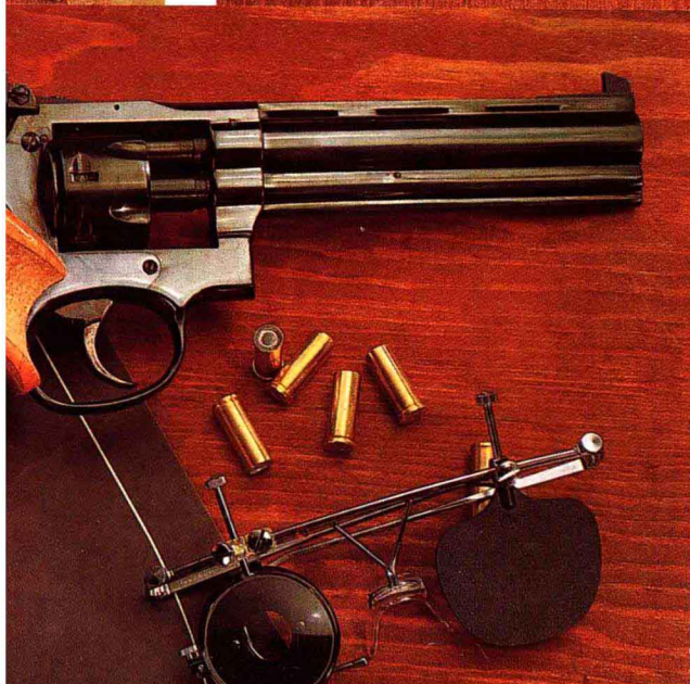
△图358 西班牙0.22英寸MXXIX式拉玛“奥林匹克”比赛转轮手枪
