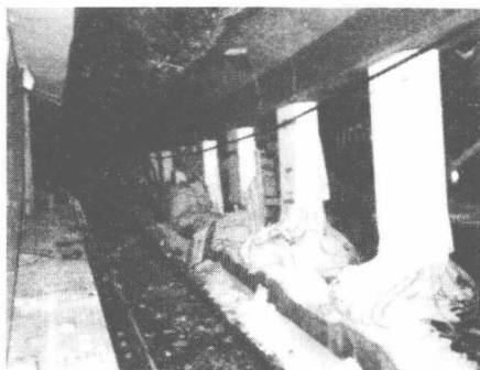
图 1-15 地下柱破坏导致路面下陷
