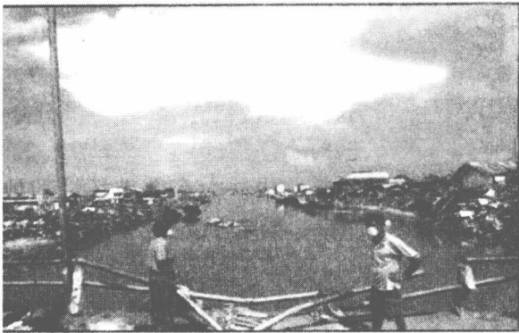
图 1-20 印度洋海啸
