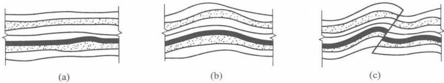
图 1-22 岩层的断裂
