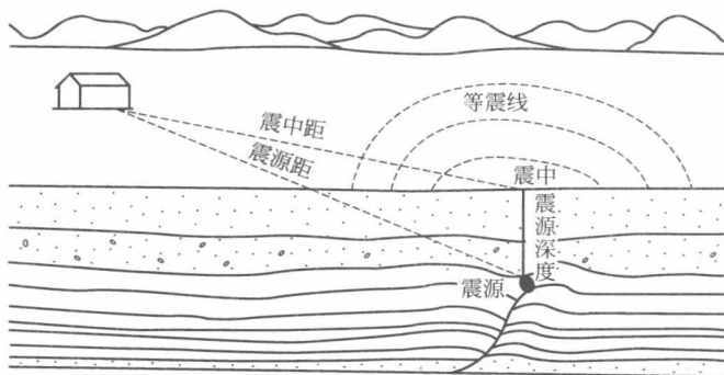
图 1-25 地震术语示意
