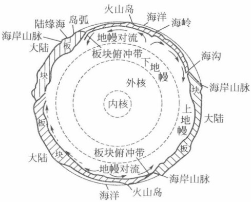
图 1-23 地球剖面图
