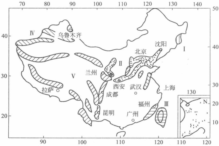
图 1-2 我国主要地震带
