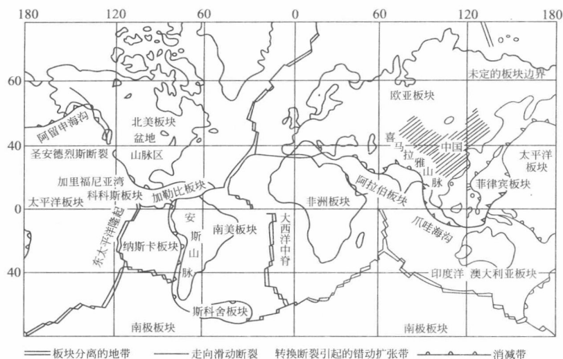
图 1-24 板块分布图
