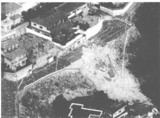
图 1-18 山体滑坡
