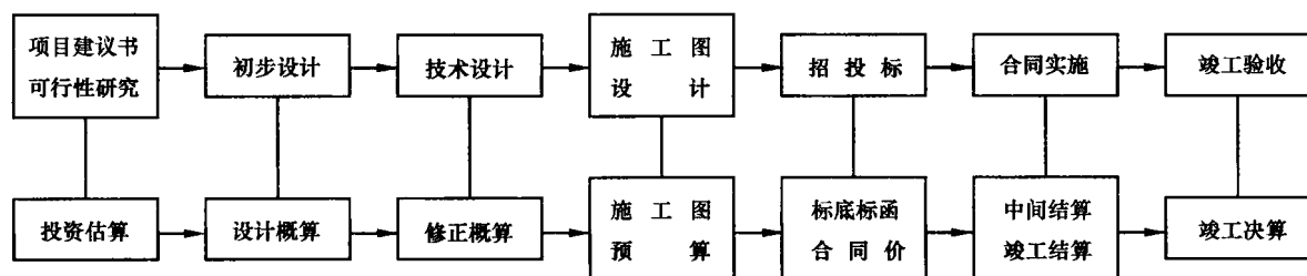
图 1-2-1 建设工程多次计价示意图
