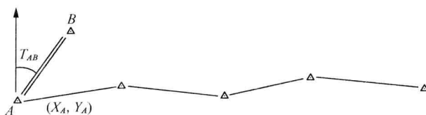
图 1-2 导线测量基本原理图
