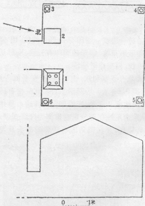
图二 辛祥墓平、剖面图
