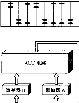
图 1.3 运算器结构示意图
