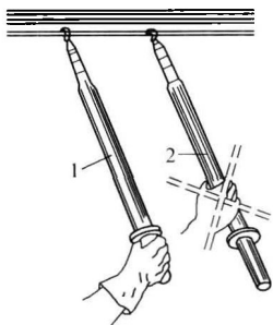
图 1-4 高压验电器使用 1—正确；2—错误
