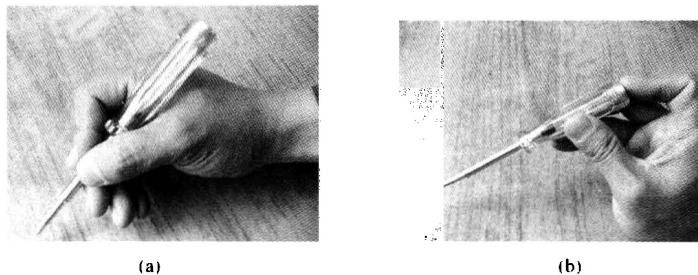
图 1-2 低压验电器的使用方法
