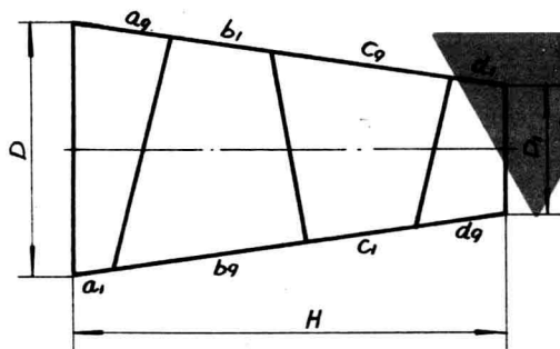
管子下料图
