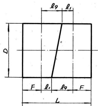
管子下料图
