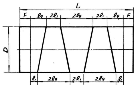
管子下料图
