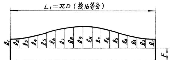
断节下料样板展开图
