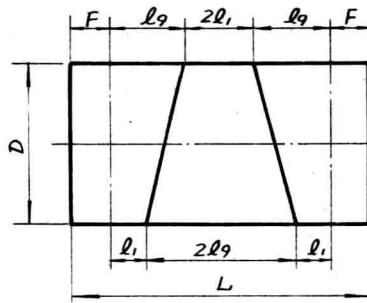
管子下料图
