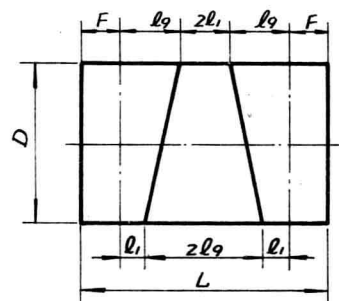
管子下料图
