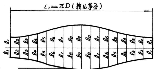
断节下料样板展开图
