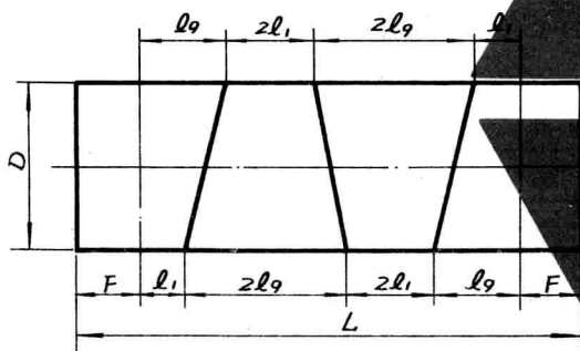
管子下料图
