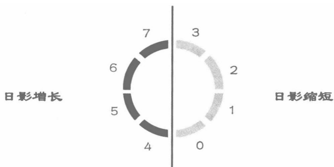
八卦的下爻
