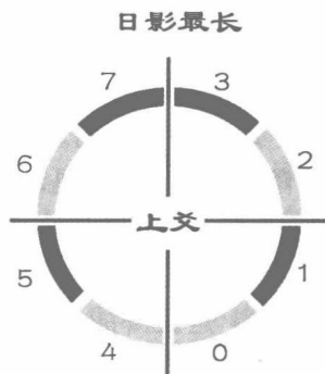
日影的变化
