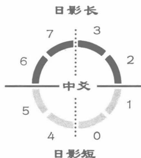
日影的变化
