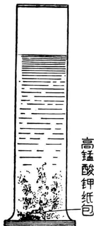
圖2 高錳酸鉀在水中的扩散
