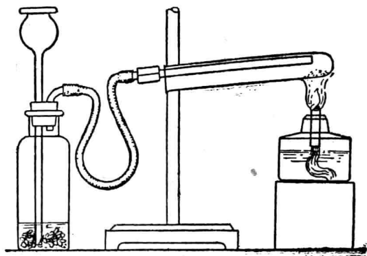
圖 5 氧化銅的還原
