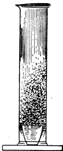
圖1 溴气在空气中的扩散
