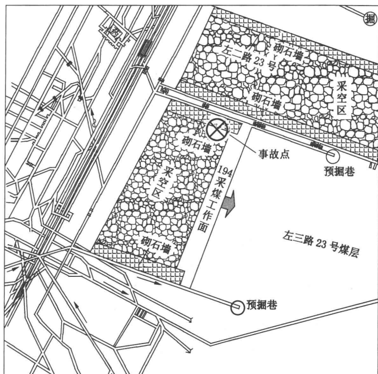
图 1-1 采空区瓦斯燃烧封闭不当引起爆炸示意图
