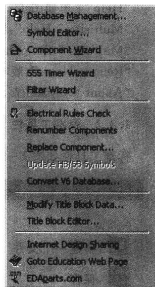
图 1-15 “Tools”菜单
