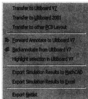
图 1-14 “Transfer”菜单
