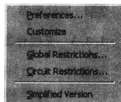
图 1-17 “Options”菜单
