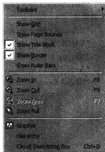
图 1-11 “View”菜单
