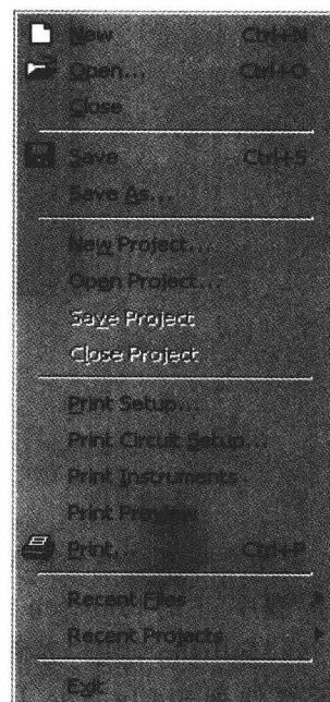
图 1-9 “File”菜单
