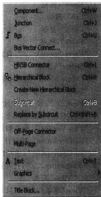
图 1-12 “Place”菜单
