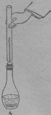
第七圖 氫焰發出樂音
