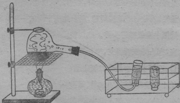
第一一圖 製造氧氣
