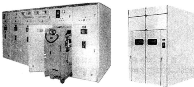
图 1.3 JYN 系列户内交流金属封闭移开式高压开关柜外形
