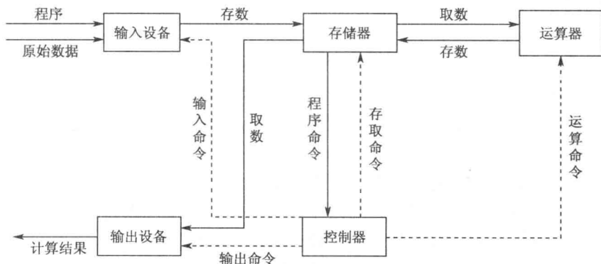
图 1.1 计算机系统基本硬件结构
