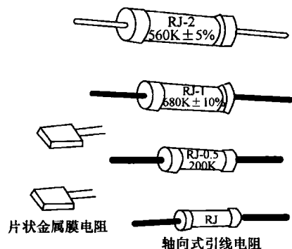
图 2.1.3 金属膜电阻器的外形
