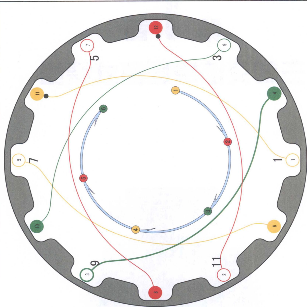
a) 嵌线图
