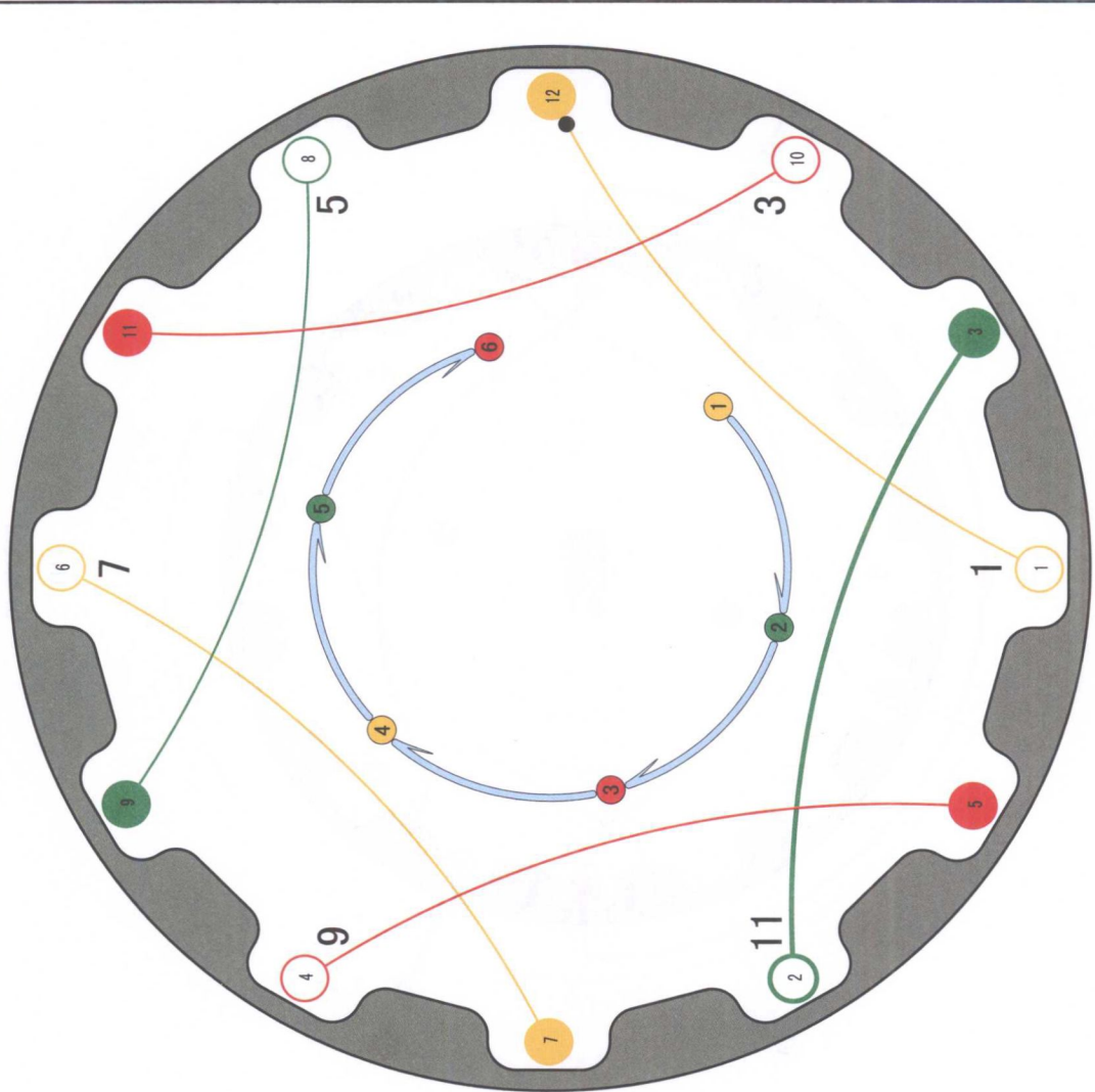
a) 嵌线图
