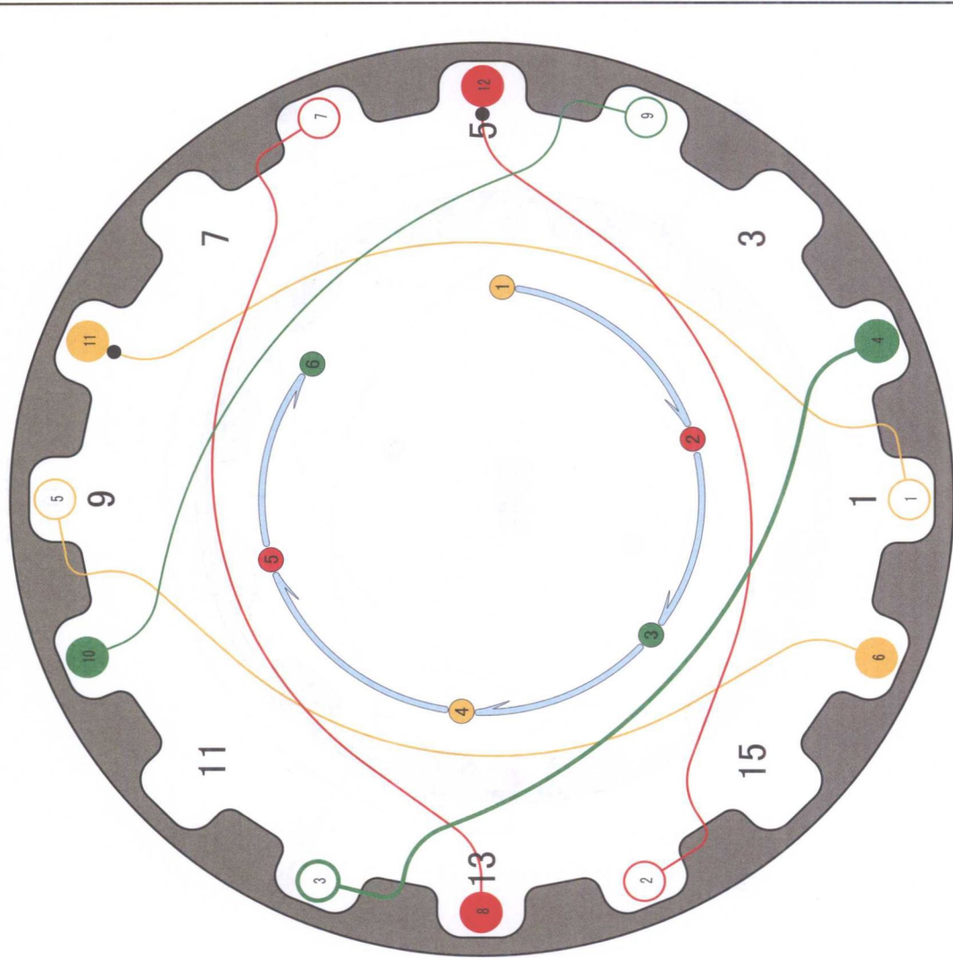
a) 嵌线图
