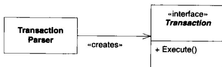
图27-1 Transaction接口
