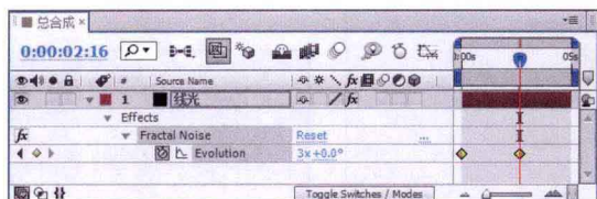
图1.8 关键帧设置
