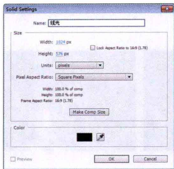
图1.4 固态层设置
