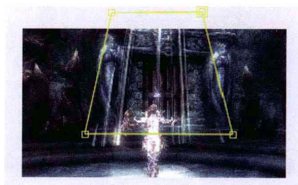
图1.13 绘制蒙版
