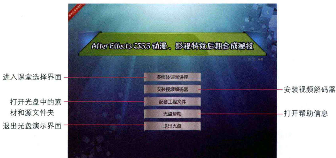
图1 主界面
