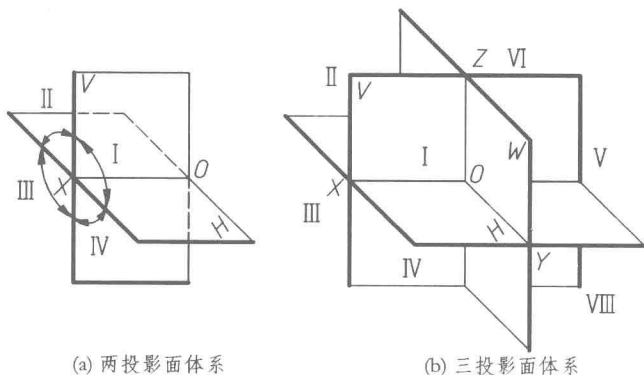
图 1-6 投影体系
