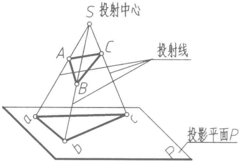
图 1-2 中心投影法
