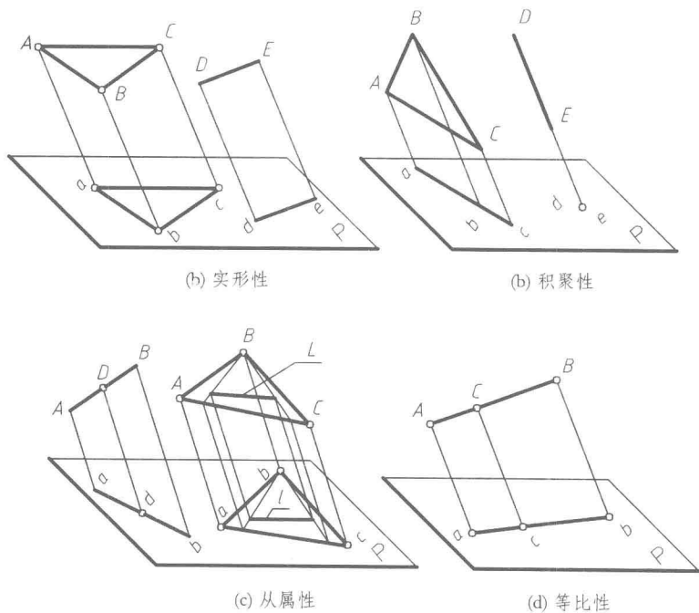
图 1-4 平行投影特性
