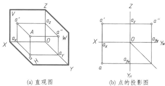
图 1-9 点的三面投影
