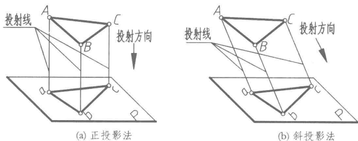
图 1-3 平行投影法
