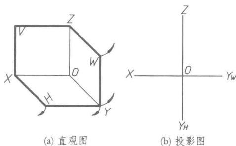
图 1-8 三面体系第 I 角
