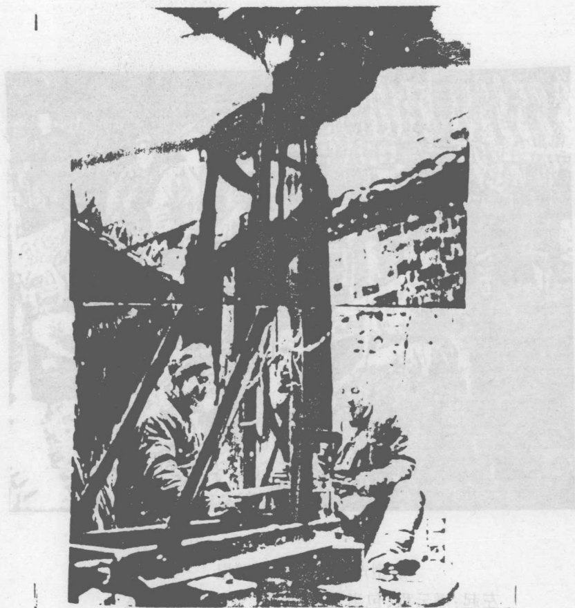
军工战士在自制的夹板锤上冲剪迫击炮弹尾翅张剑中(右)
