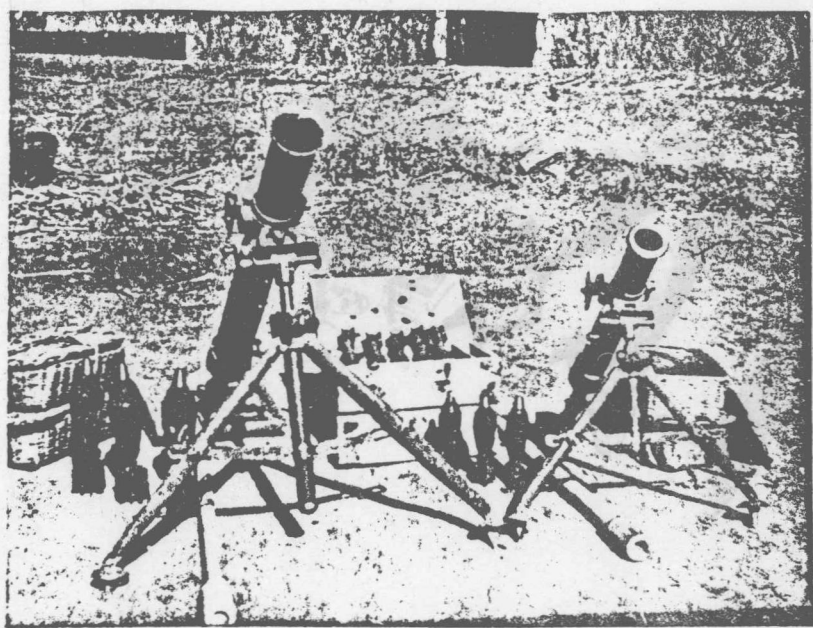
迫击炮、炮弹和炮刷。左 73 毫米，右 52 毫米，竹篮是代替木箱作炮弹包装用
