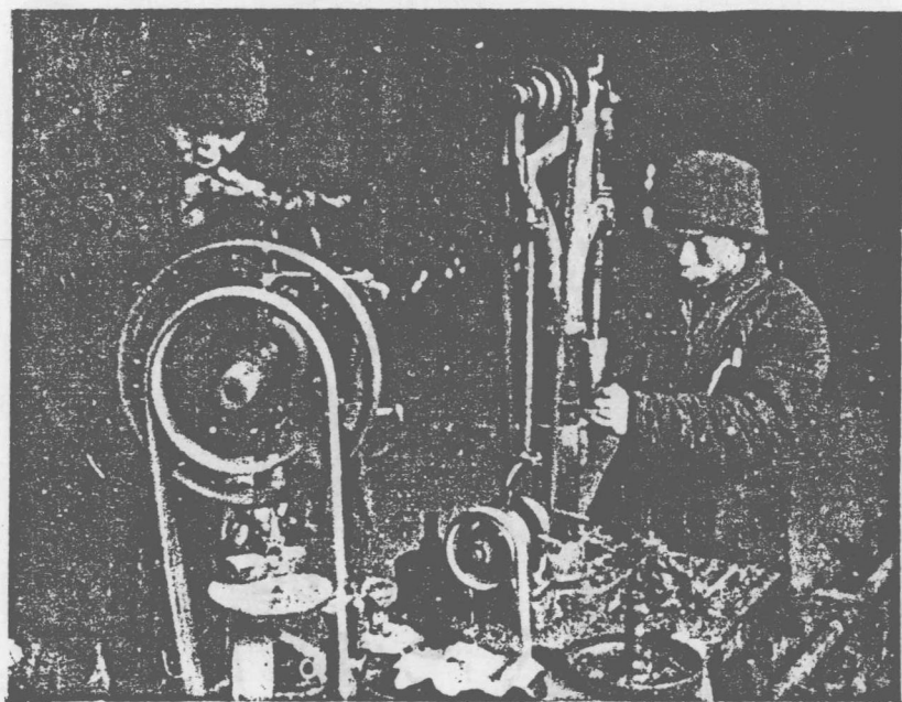
钻工 左:陆叶坤,右:戴祖芳 右边钻床是军工部仿制的, 左边钻床是手摇动改成柴油机动力的
