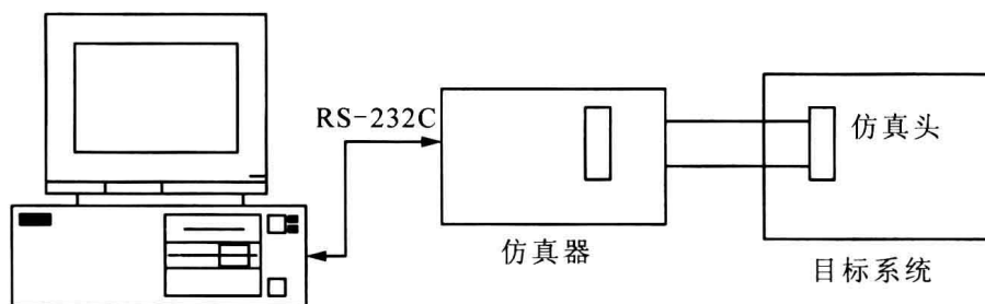
图 1-1 常见开发系统的一般结构
