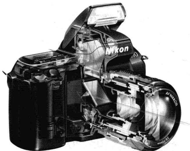
照片 21 尼康 F70 照相机剖面图
