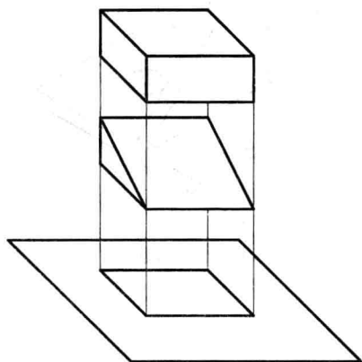
图 1-14 单面投影
