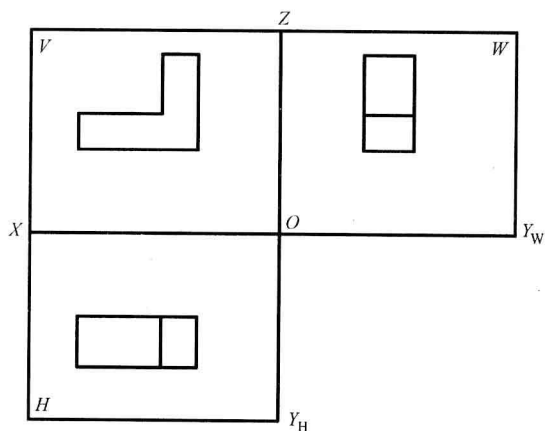
图 1-18 三面投影图
