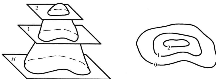
图 1-13 标高投影图
