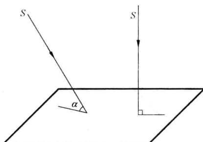
图 1-4 斜投影、正投影
