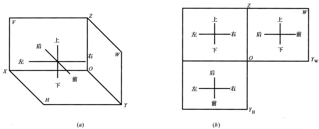
图 1-20 方向的确定
