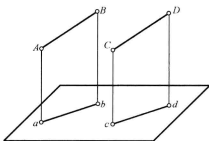
图 1-7 平行性
