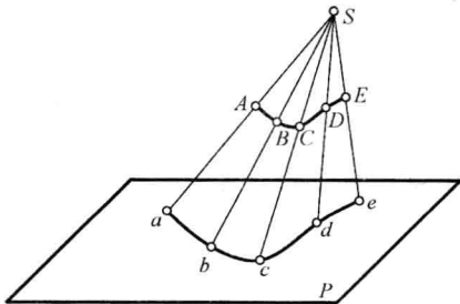
图 1-2 中心投影
