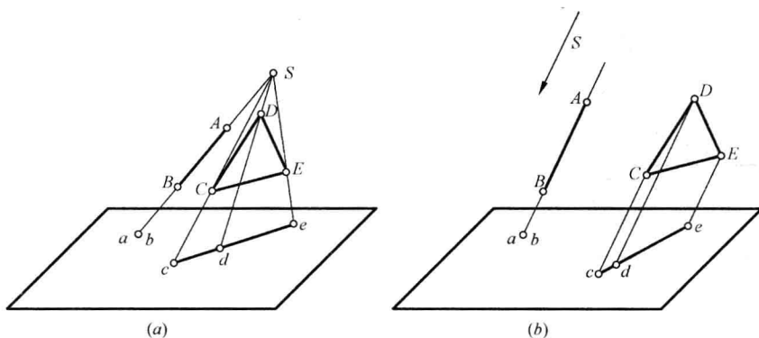
图 1-5 积聚性
