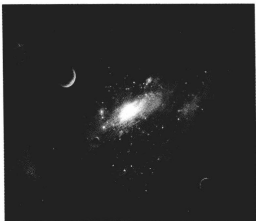
◆宇宙源于道
