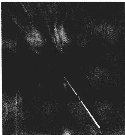
◆飞矢不动
