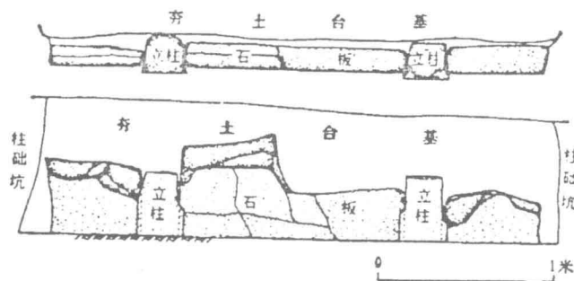
图六 1号院落F1夯土台两侧包边 石构件平(上)、立(下)面局部图
