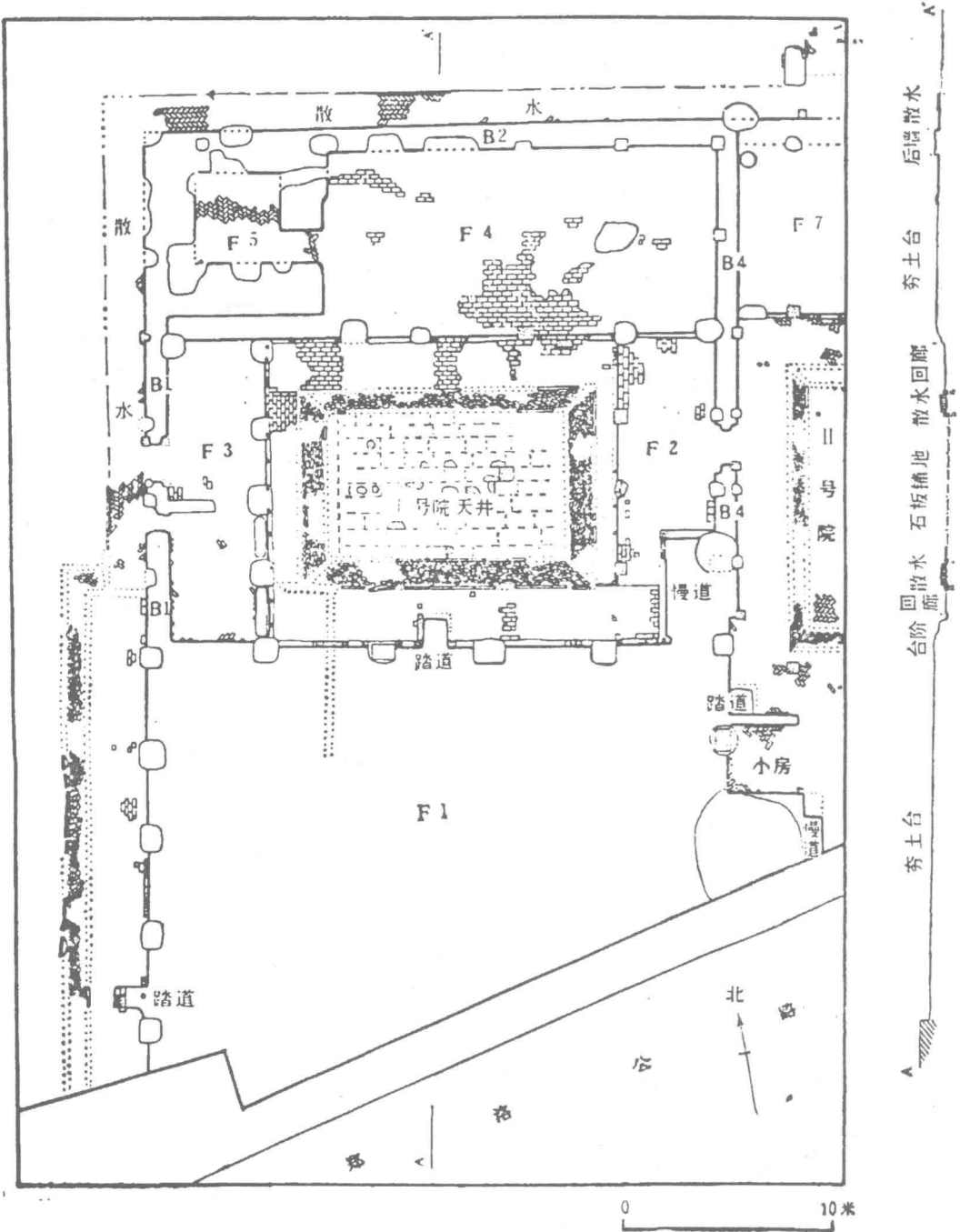
图四 I号院落平、剖面图
