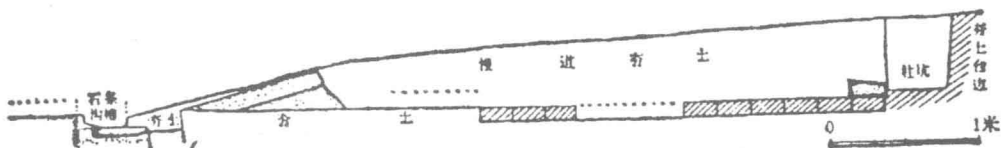
图五 I号院落F1东北角慢道立面图
