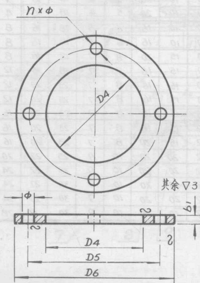
7-法兰盘
