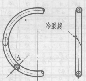
4-橡皮条
