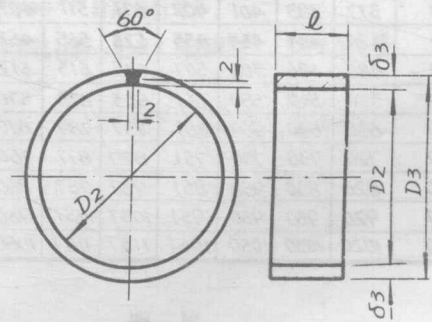
8-短管
