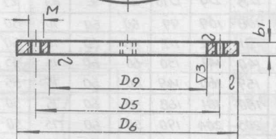
9-翼盘
