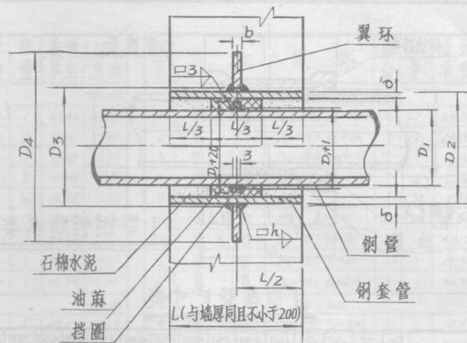
IV型刚性防水套管
