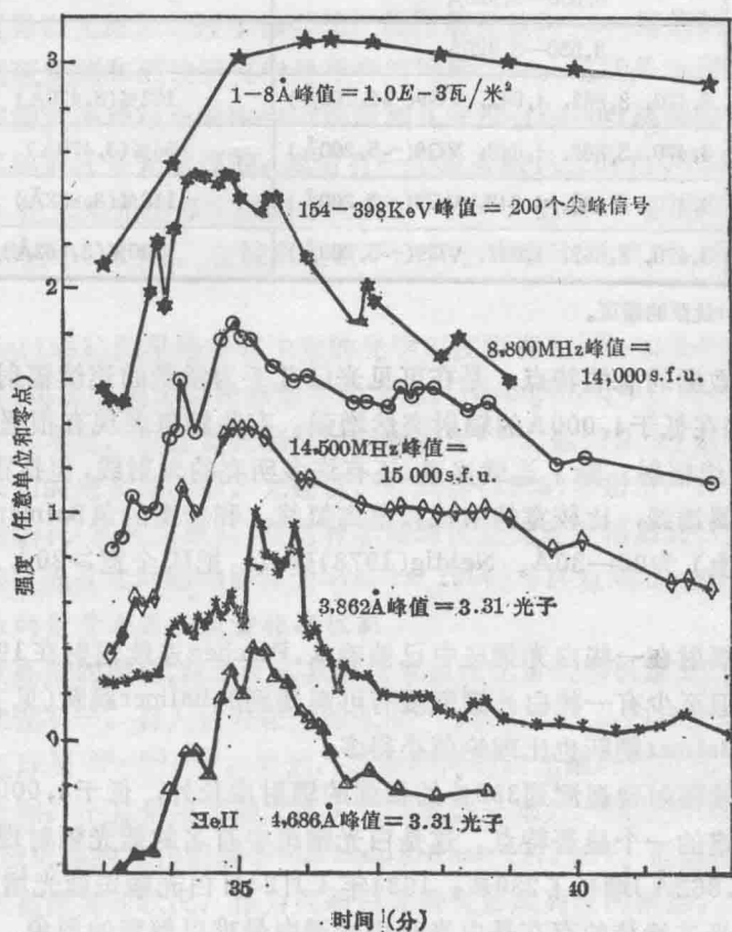
图2 1984年5月20日白光耀斑光变曲线 [14] 。
