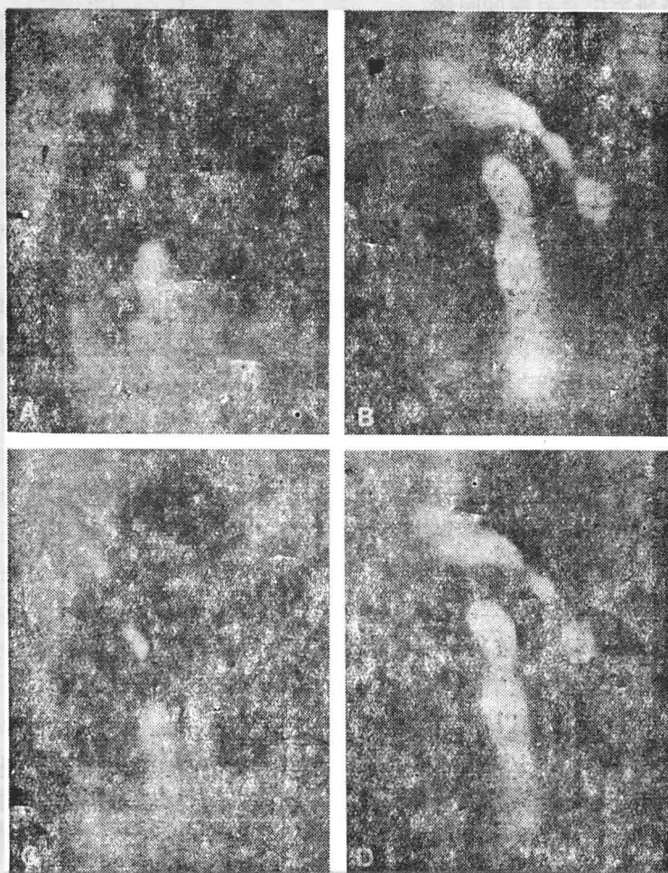
图1. 1984年4月24日白光耀斑宽带单色象。
