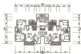
四层平面图
