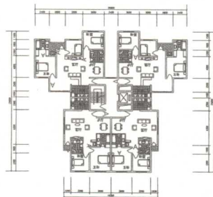
三层平面图
