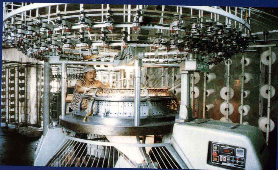
会纺集团针织大圆机
