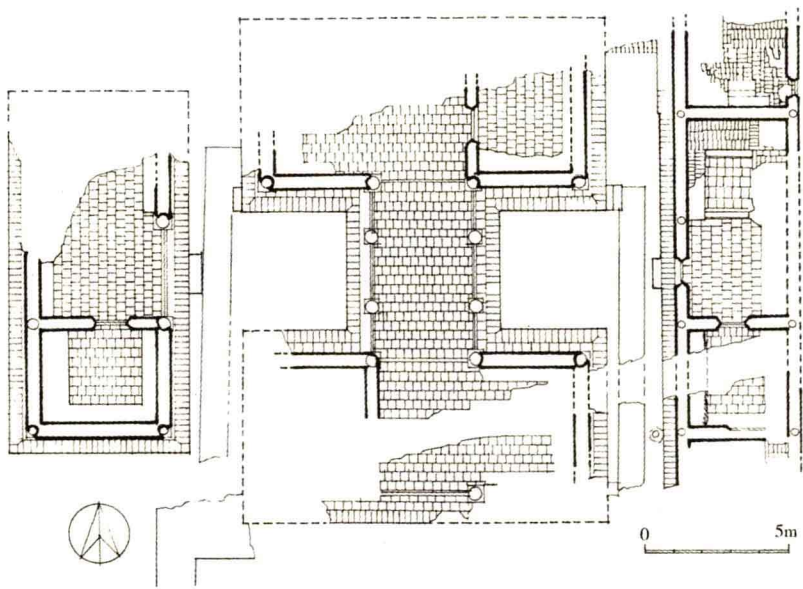
图 1-7 北京北城后英房胡同元代住宅复原平面图
