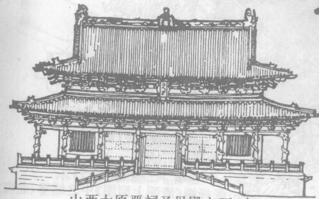
山西太原晋祠圣母殿立面(宋)
