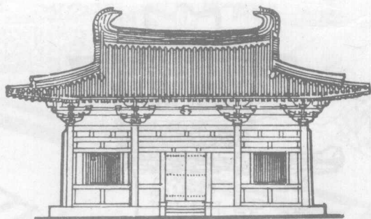
南禅寺正殿(唐)
