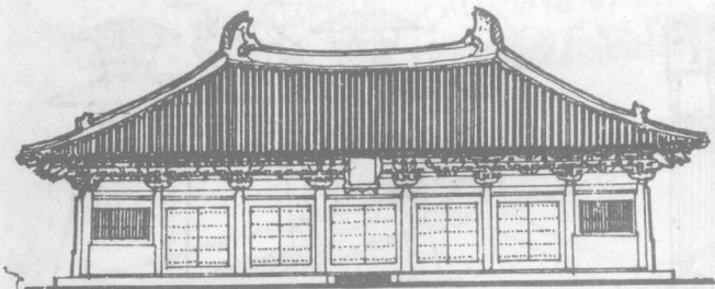
佛光寺大殿(唐)
