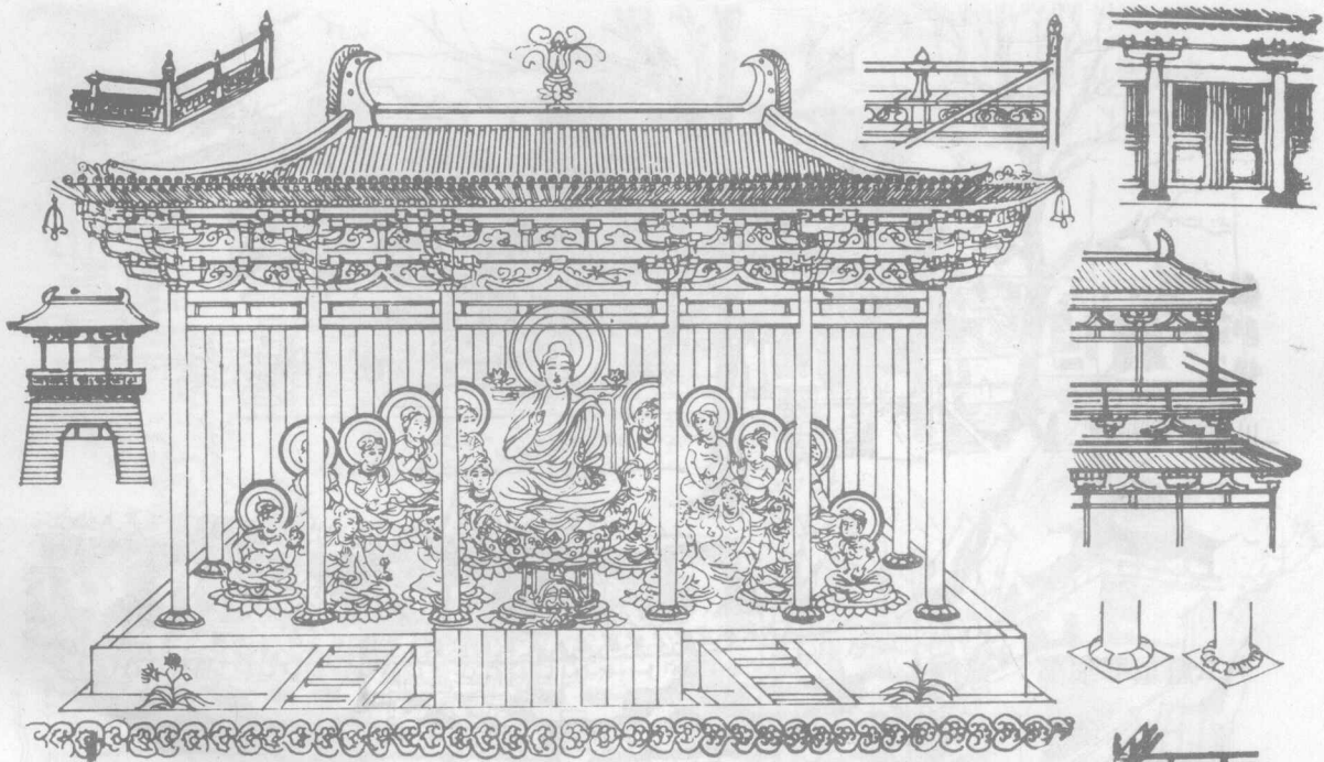
唐代建筑细部
