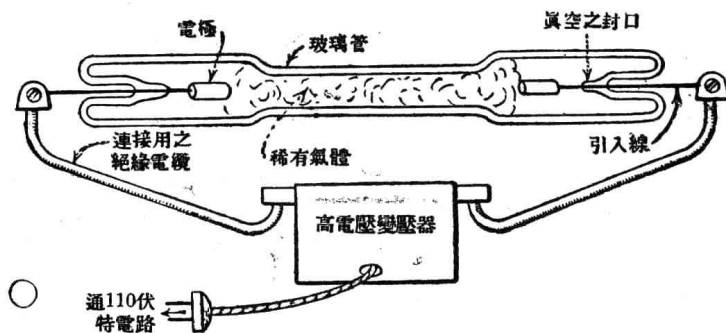
第一圖 霓虹管及變壓器之連接簡圖。
