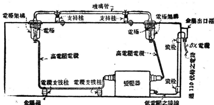
第二圖 箱式氬燈之全圖(即示霓虹管，變壓器及電纜等之地位)。
