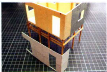
12 對應木屋外牆，剝出門和窗的空位。
