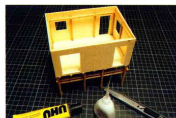
05 裝上四塊立面木板。
