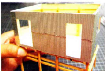
13 把切割好的波浪紋塑膠板黏貼在外牆上。
