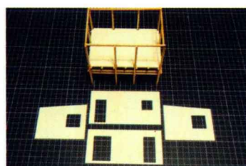
03 另將木板削出成屋的立面，門和窗的位置需削空。
