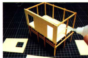
04 用超能膠將立面木板黏在屋的支架上。
