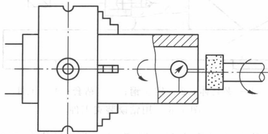
图 1-4 直接找正法加工套筒零件
