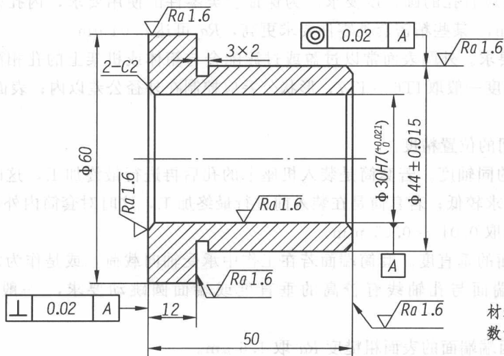
图 1-1 轴承套零件图
