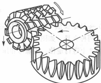
图 1-3 滚齿加工
