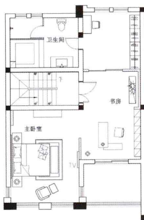
三层平面布置图
