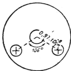
图2 氧原子电子云内氢核子的潜入
