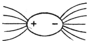
图1 水的极性分子（偶极）
