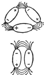
图3 水偶极形成的贰聚水和叁聚水
