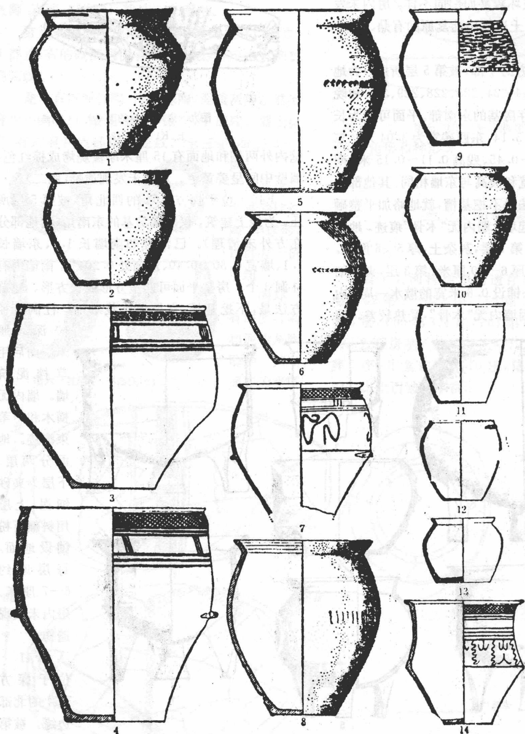
图一 大河村类型陶罐
