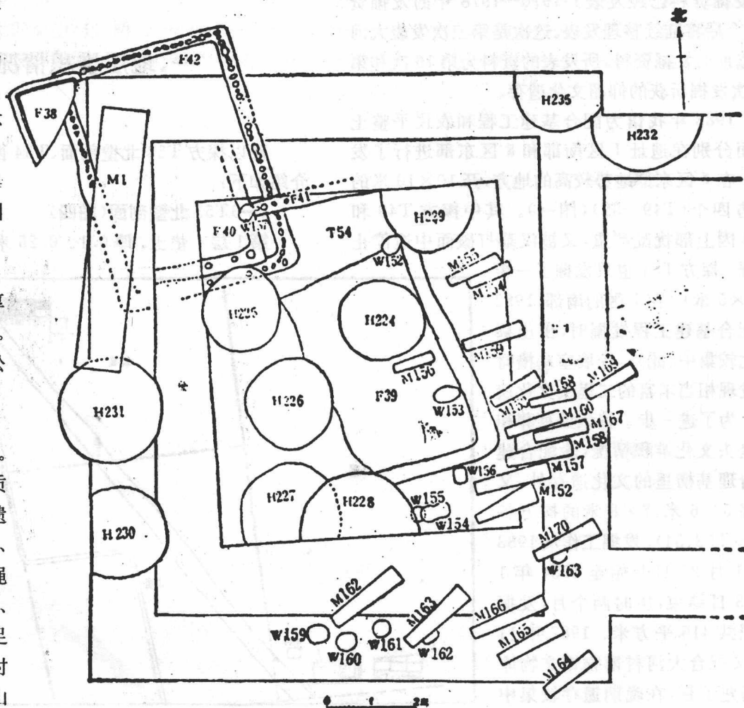
图二 T54 及西展厅基槽遗迹分布图(M1 为汉墓,图中除仰韶文化遗迹外还有部分龙山文化遗迹,报告另发)
