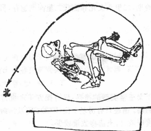
图七 H218 平、剖面图(1/25)
