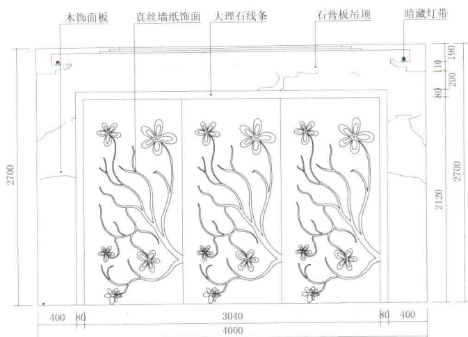
餐厅背景立面图
