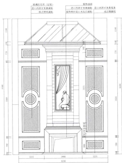
餐厅背景立面图
