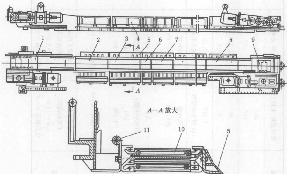
图 1-3 SGB-630/150 型刮板输送机总装图
