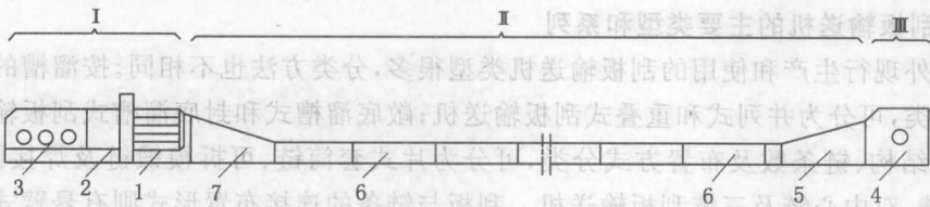
图 1-1 刮板输送机的组成
