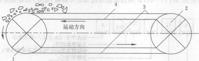
图 1-2 刮板输送机工作原理示意图
