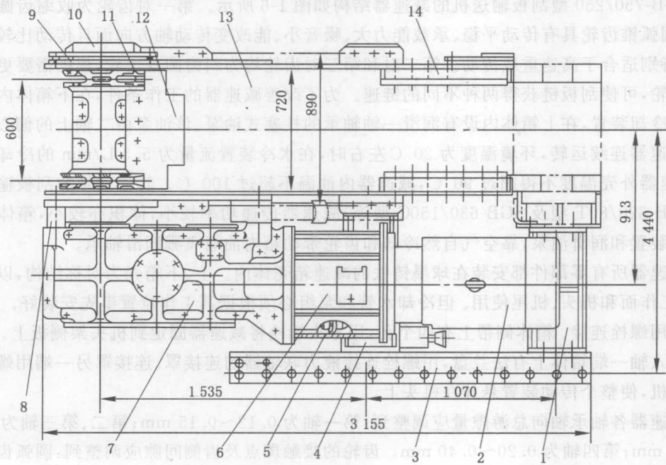
图 1-5 SGB-750/250 型刮板输送机机头部
