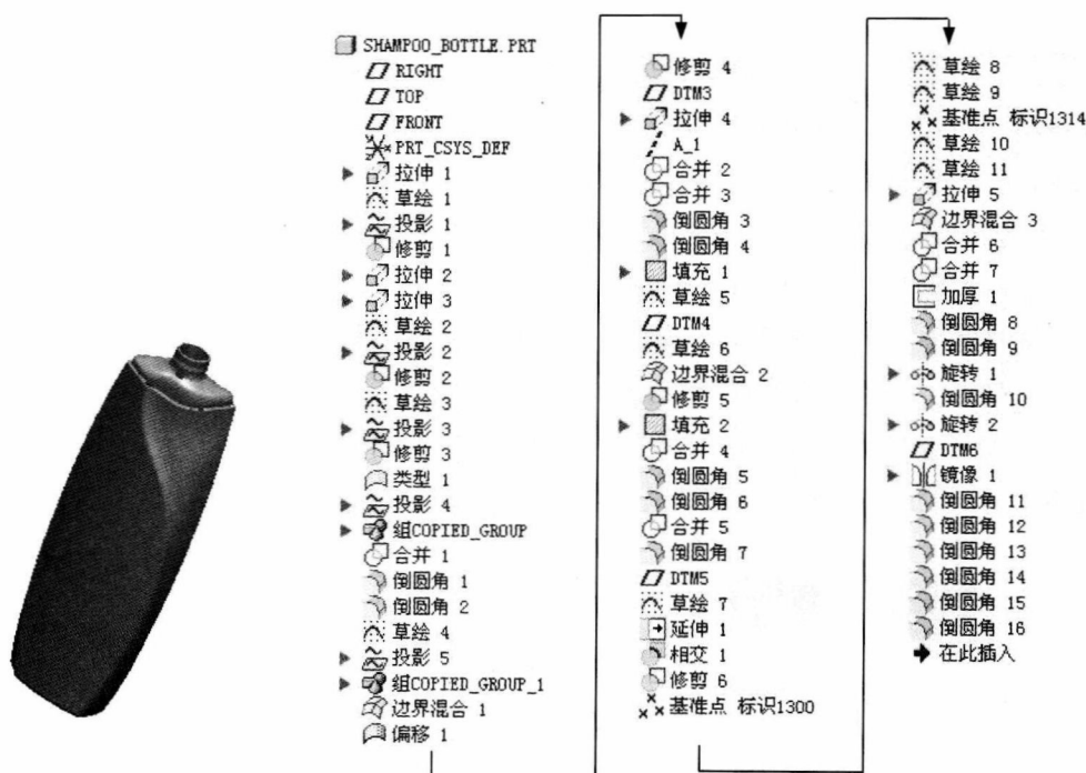
图 1.1 零件模型及模型树
