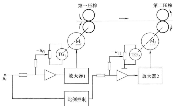
图 1-1-6 造纸机分部传动闭环控制系统
