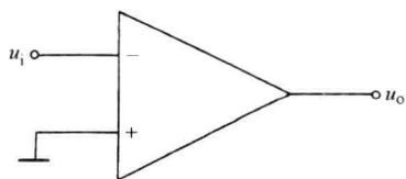
图 1-1-8 运算放大器
