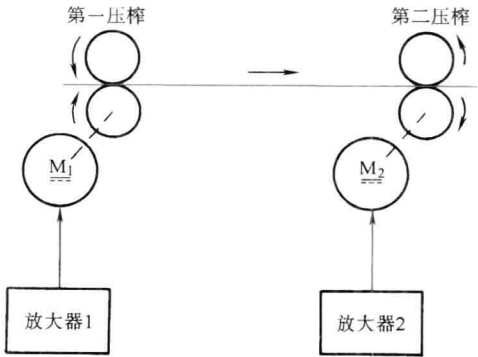
图 1-1-5 造纸机分部传动系统
