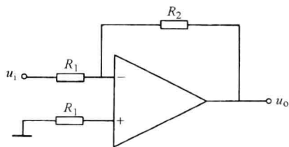
图 1-1-9 接成闭环电路的运算放大器
