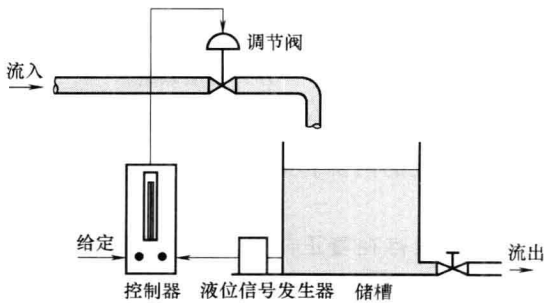
图 1-1-4 液面闭环控制系统
