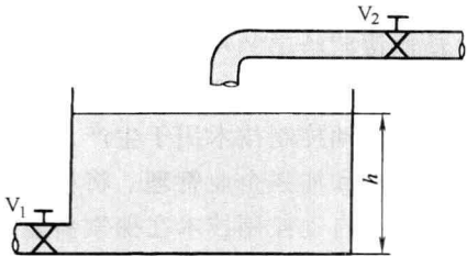
图 1-1-3 液面开环控制系统
