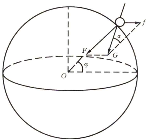
重力 G 与 引力 F 和离心 力 f 之间的关 系示意图
