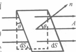
图 11-1-2 通过 dS 的电通量
