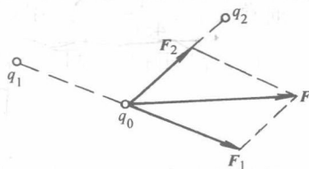
图 11-2-2 电力叠加原理
