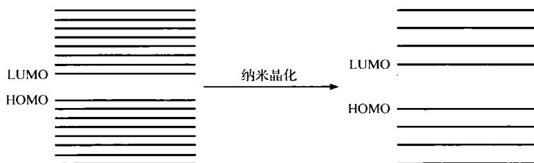
图 1.1 金属的量子尺寸效应示意图
