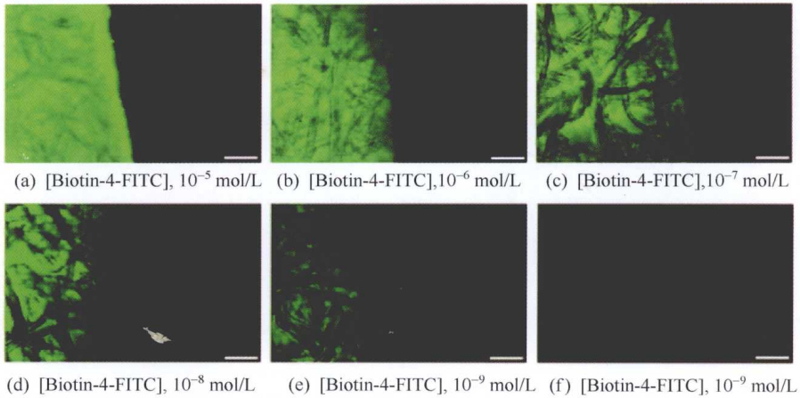
图 12-24 链酶亲和素修饰的纤维素材料结合荧光标记的生物素后的荧光显微照片。每张荧光显微照片的左部分为荧光标记的不同浓度的生物素与样品结合后的照片,右部分为不做任何修饰的滤纸纤维素材料的荧光显微照片。标尺长度为 100\ \mu\text{m}
