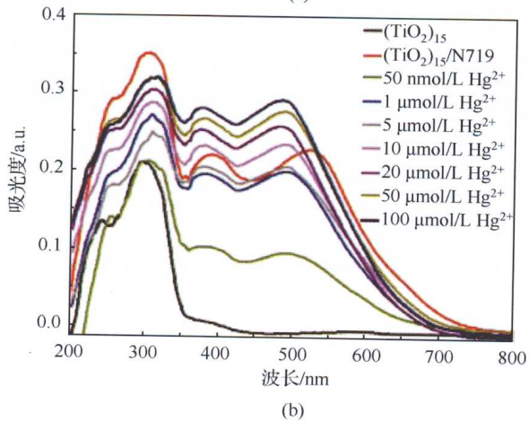
图 12-22 N719 修饰的滤纸对 \text{Hg}^{2+} 的传感效果
