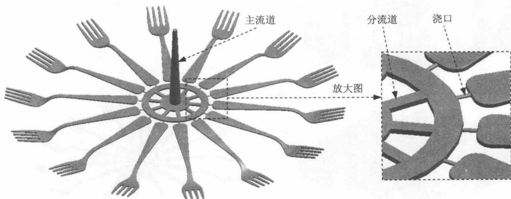
图 1.1.5 浇注系统
