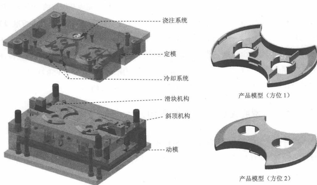
图 1.1.6 模架设计
