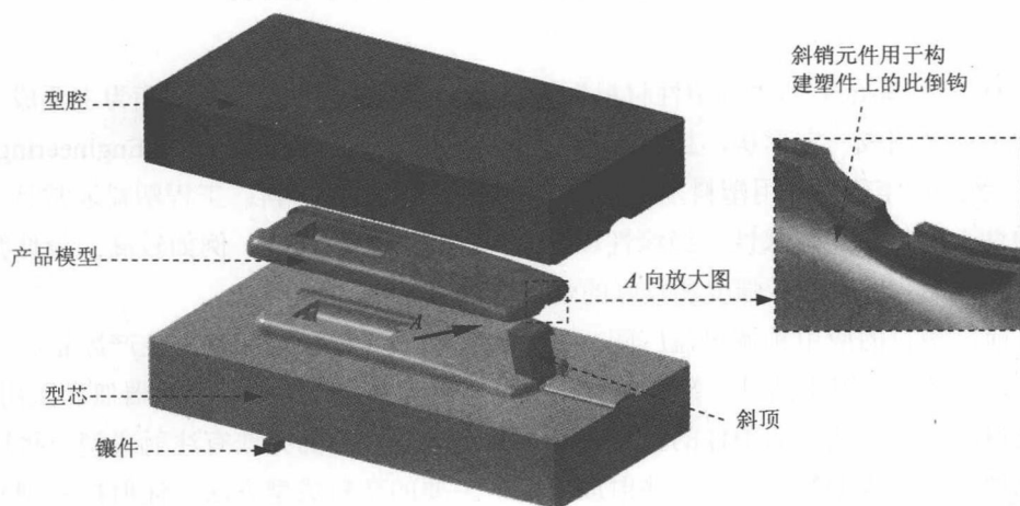
图 1.1.3 塑件成型元件 (带斜顶)
