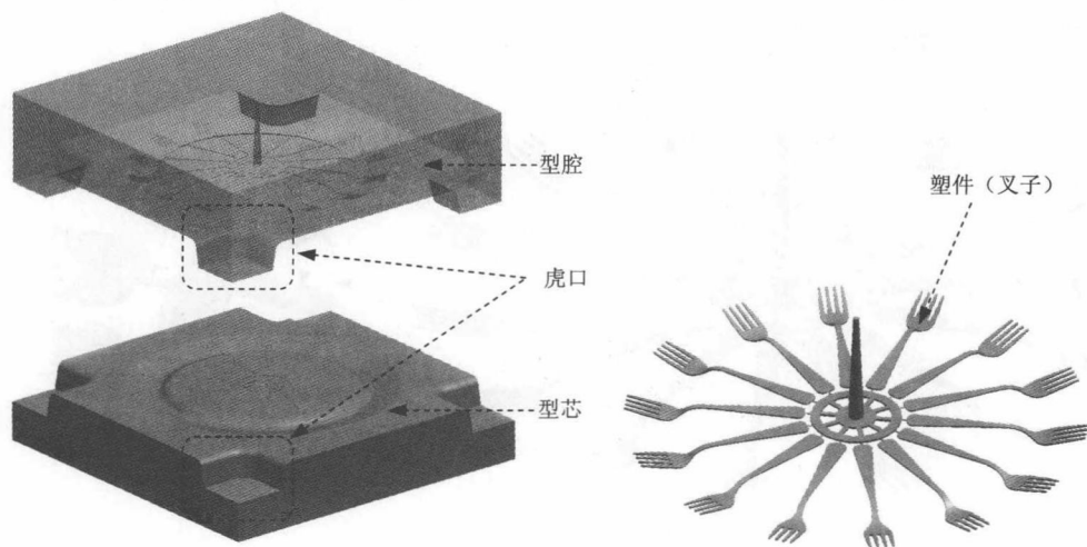
图 1.1.7 在“零件设计”工作台下进行模具设计
